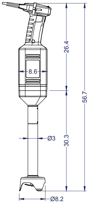
Vista Elevación
