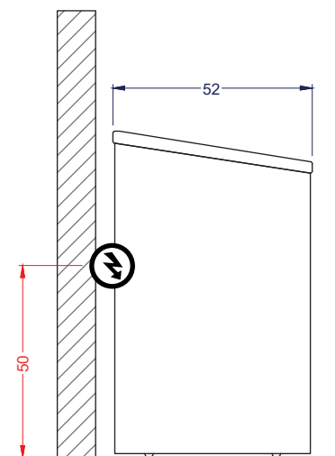
Vista Izquierda
