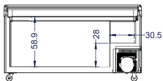
Vista Elevación
