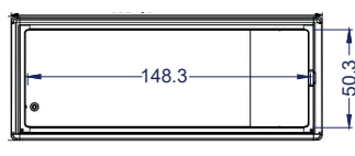
Vista Izquierda
