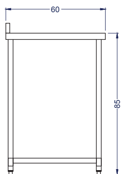
Vista Izquierda
