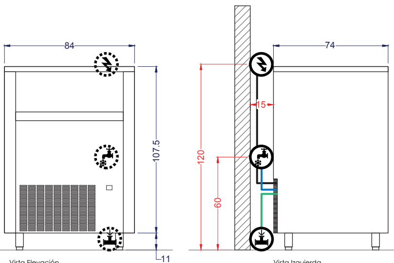
Vista Elevación
