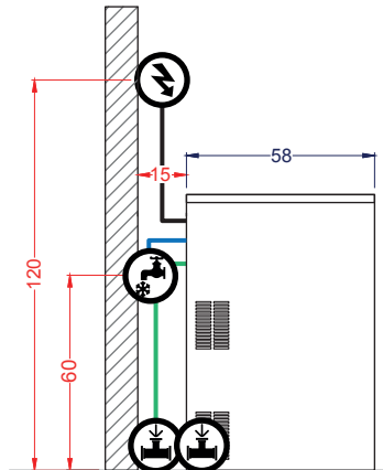
Vista Izquierda
