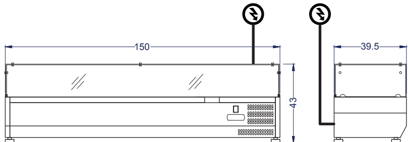
Vista Elevación
