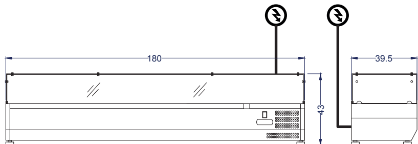
Vista Elevación
