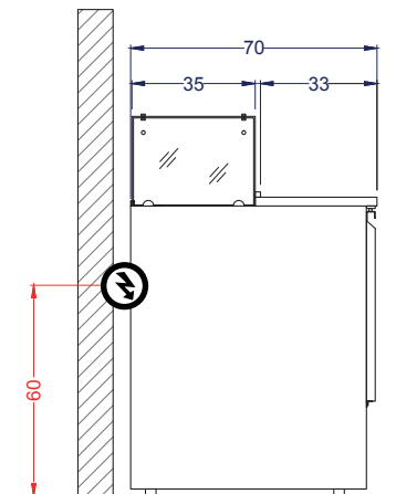
Vista Izquierda
