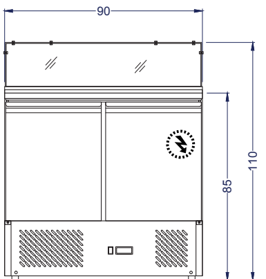
Vista Elevación
