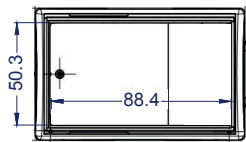
Vista Planta
