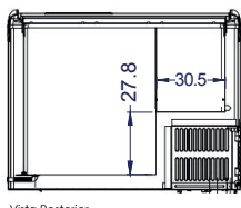
Vista Posterior
